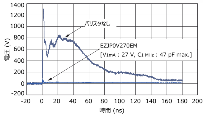
[静電気抑制波形]
