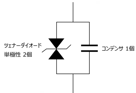
[積層バリスタの等価回路]
