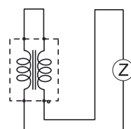
(B) ディファレンシャルモード
