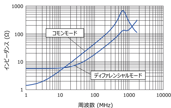
(B) ディファレンシャルモード
