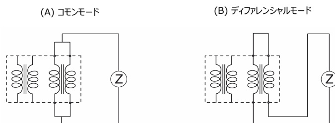
● 測定回路
