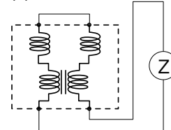
(C) デファレンシャルモード
