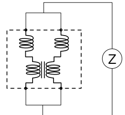
(B) コモンモード
