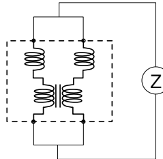
(B) コモンモード
