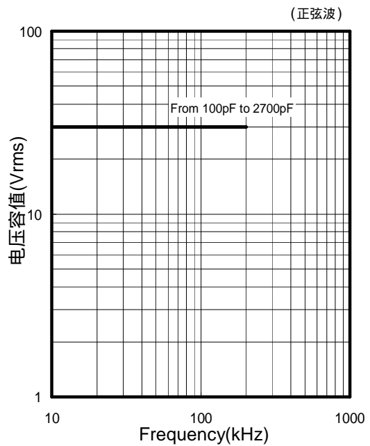
电压容值
