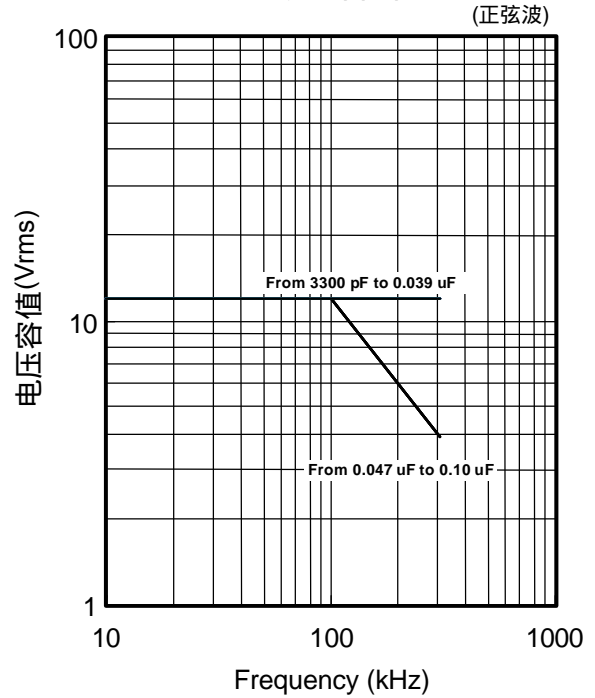
电压容值
