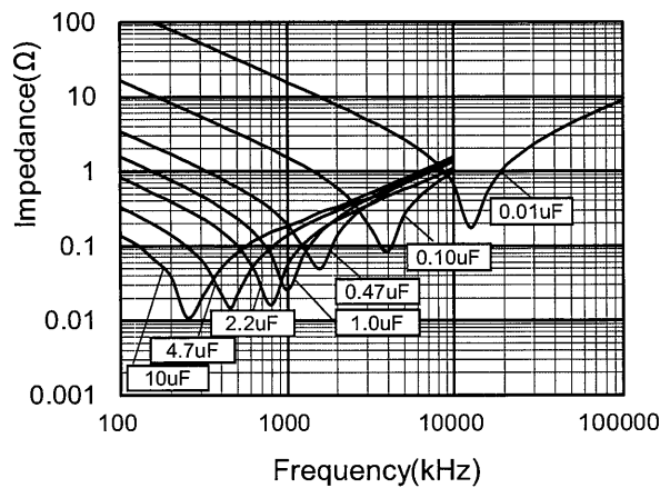
阻抗特性
