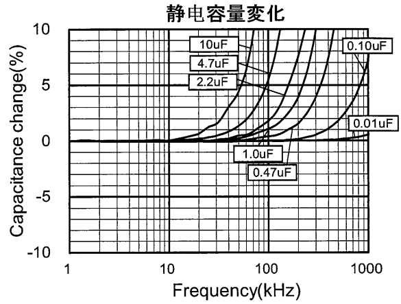
频率特性
