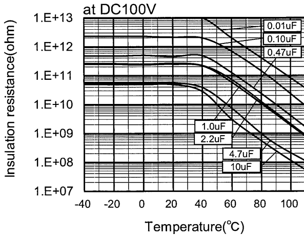
绝缘电阻变化
