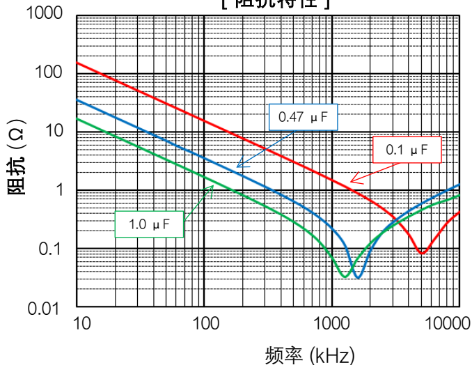
[ 阻抗特性 ]
