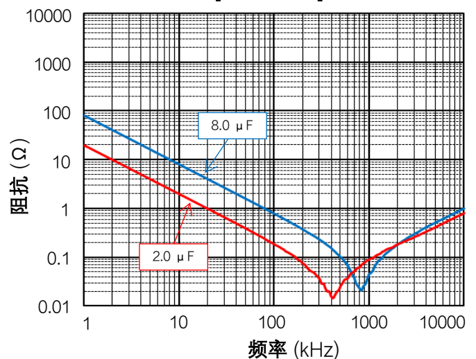
[ 阻抗特性 ]
