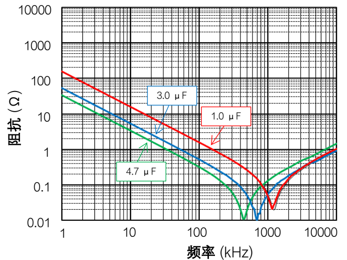
[ 阻抗特性 ]
