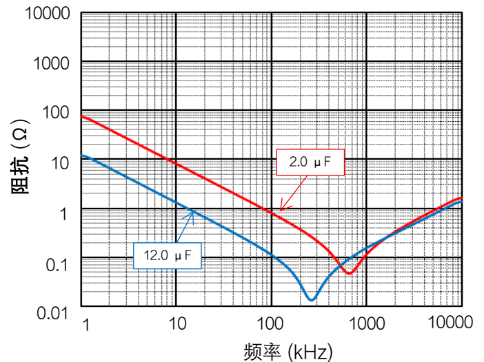
[ 阻抗特性 ]
