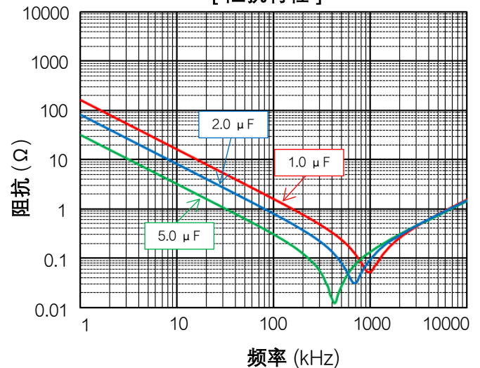
[ 阻抗特性 ]
