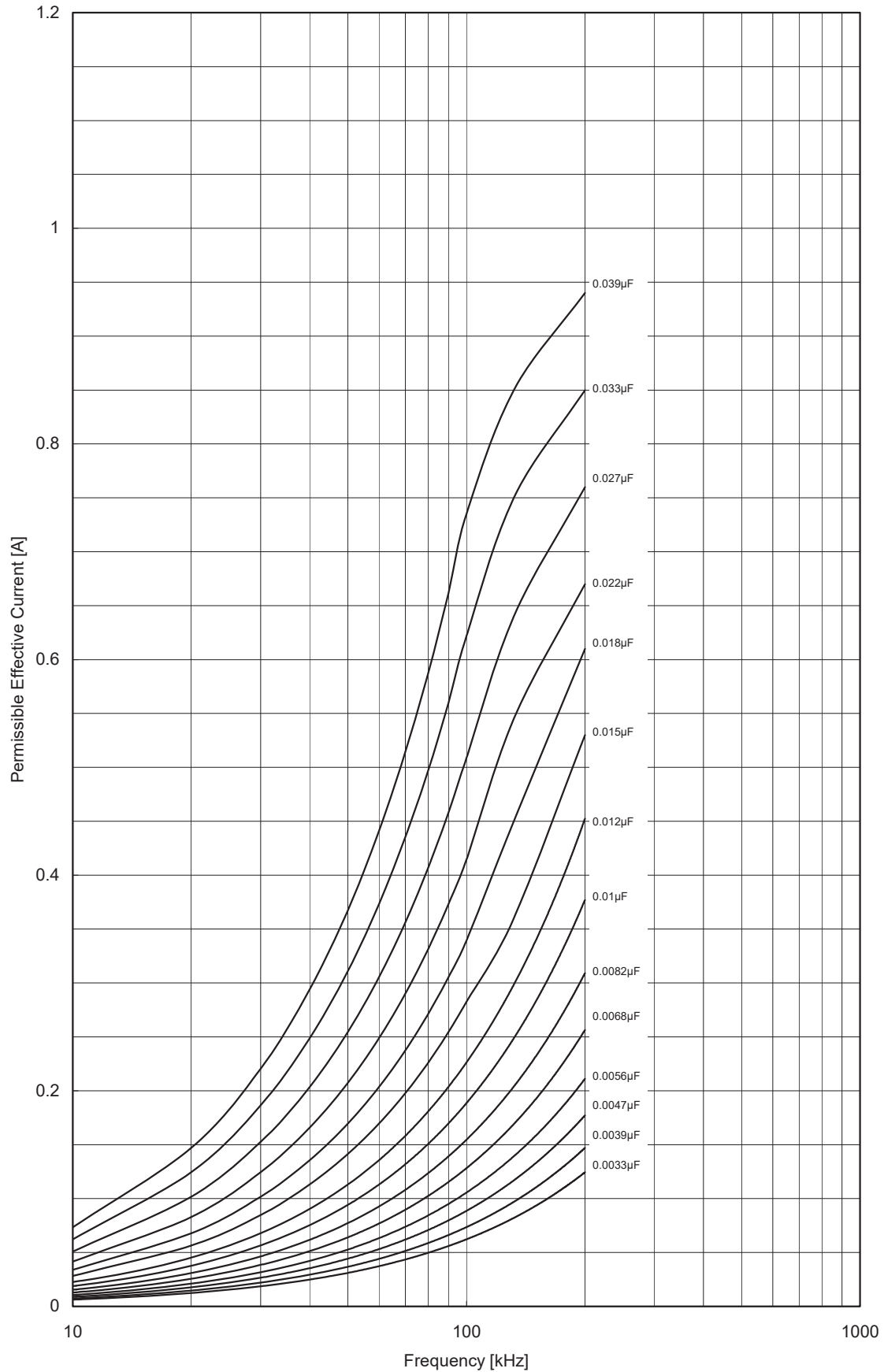
Fig. 5 周波数別許容電流値 ECHU1H(X):(0.0033 \mu F~0.039 \mu F) 測定条件:正弦波
