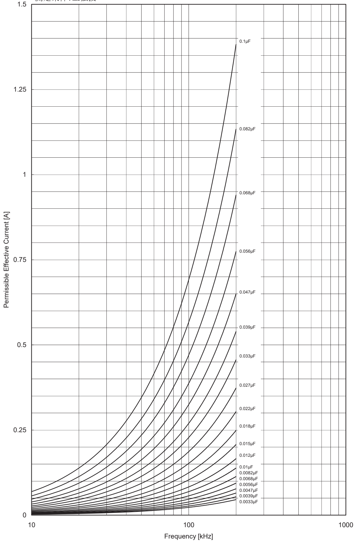
Fig. 3 周波数別許容電流値 ECHU1C(X):(0.0033 \mu F \sim 0.10 \mu F) 測定条件:正弦波
