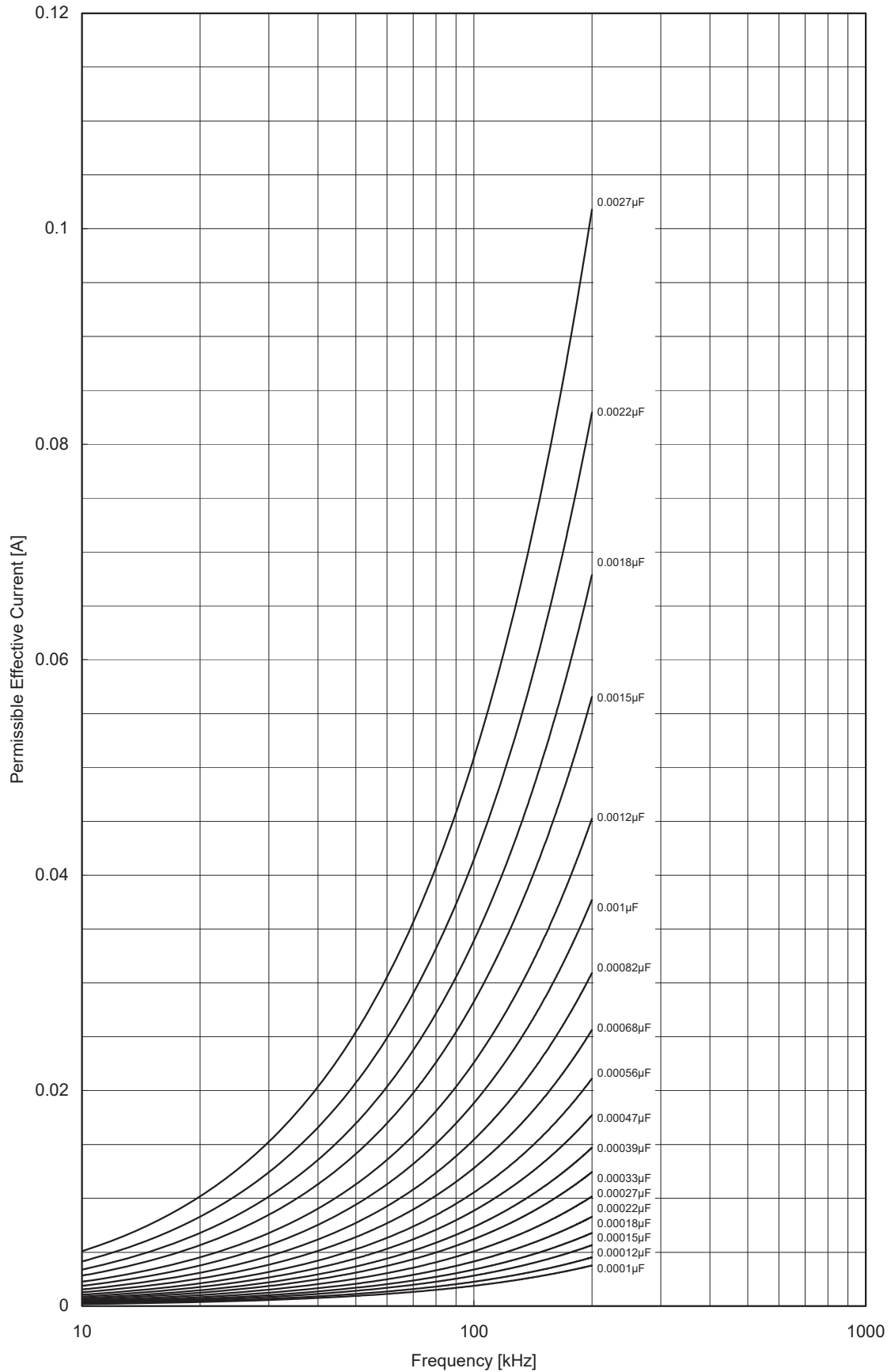
Fig. 4 周波数別許容電流値 ECHU1H(X):(0.00010 \mu F~0.0027 \mu F) 測定条件: 正弦波
