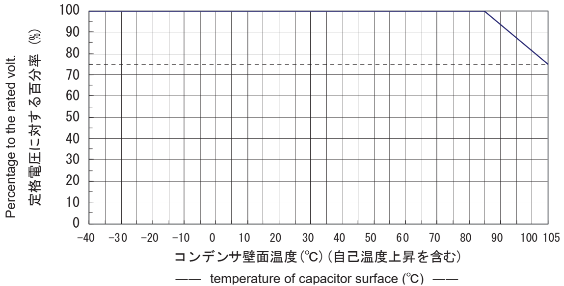
図-1 使用温度に対する定格電圧の軽減曲線
